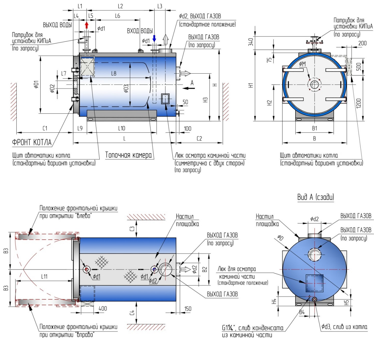
Рис. 1. Габаритные и установочные размеры котлов «ТУРБОТЕРМ»
