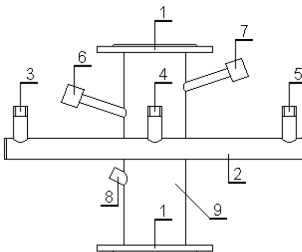
Рис. 2. Вертикальный отвод для установки группы безопасности.
